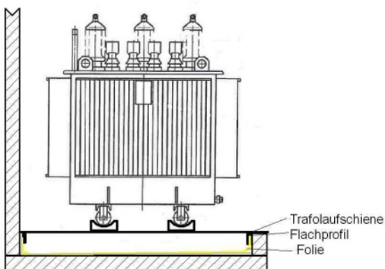
Typ 1: Boden ist eben und Raum angemessen zum Trafo
