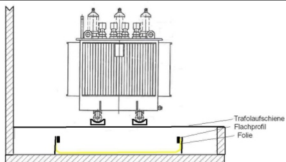
Typ 2: Boden ist eben und Raum viel größer als Abmessung Trafo
